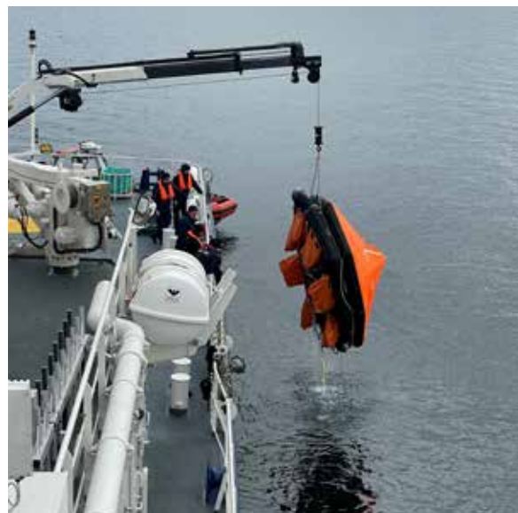
Die Rettungsinsel wird mit dem Bordkran gefischt.
